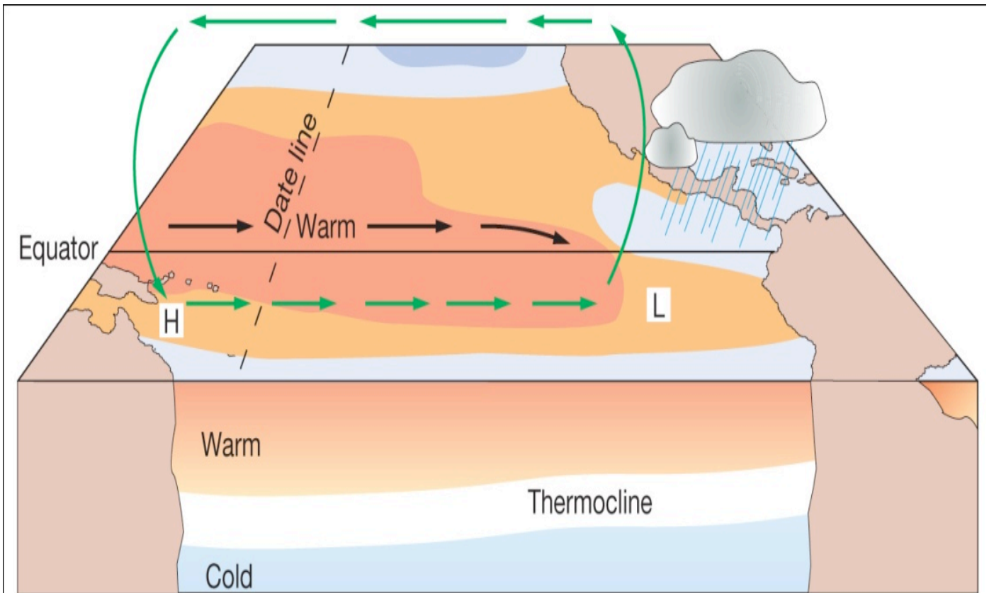
(b) El Niño conditions (strong)
