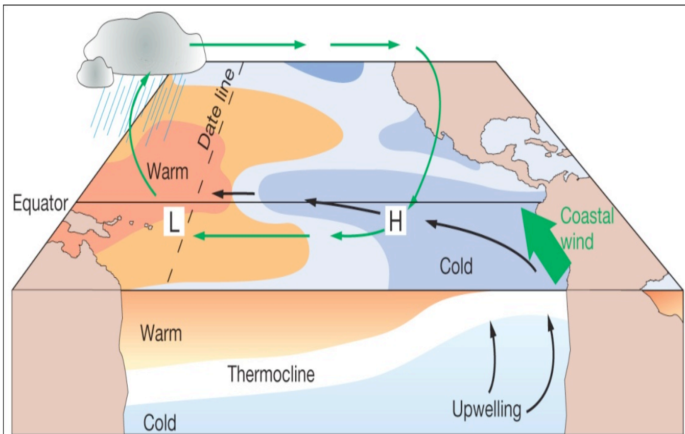
(c) La Niña conditions
